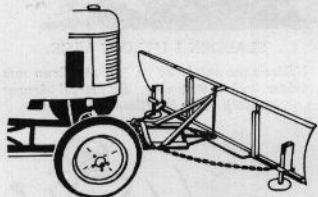
På bladets baksida finns 2 st. ställbara tallriksmedar av 12 mm tjock stålplåt.
