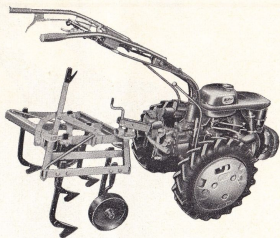
Kultivator med dubbelparallelogram.
