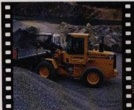
Det nya lastaggregatet TP-linkage gör Volvo BM L50B till en smidig och effektiv skopplastare. TP-linkage ger högt brytmoment inom hela lyftområdet.
