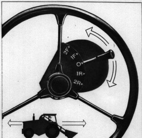
Snabb fram- och backkörning genom växelväjljare
