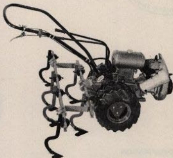
Cliotrac 21 med universalfäste och kultivator typ J 36d/2
