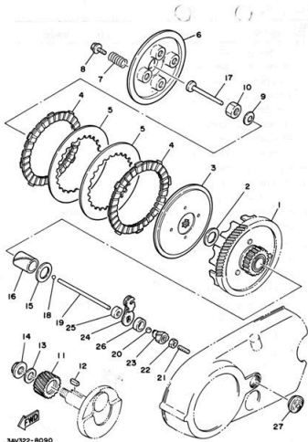
FIG. 9 CLUTCH
